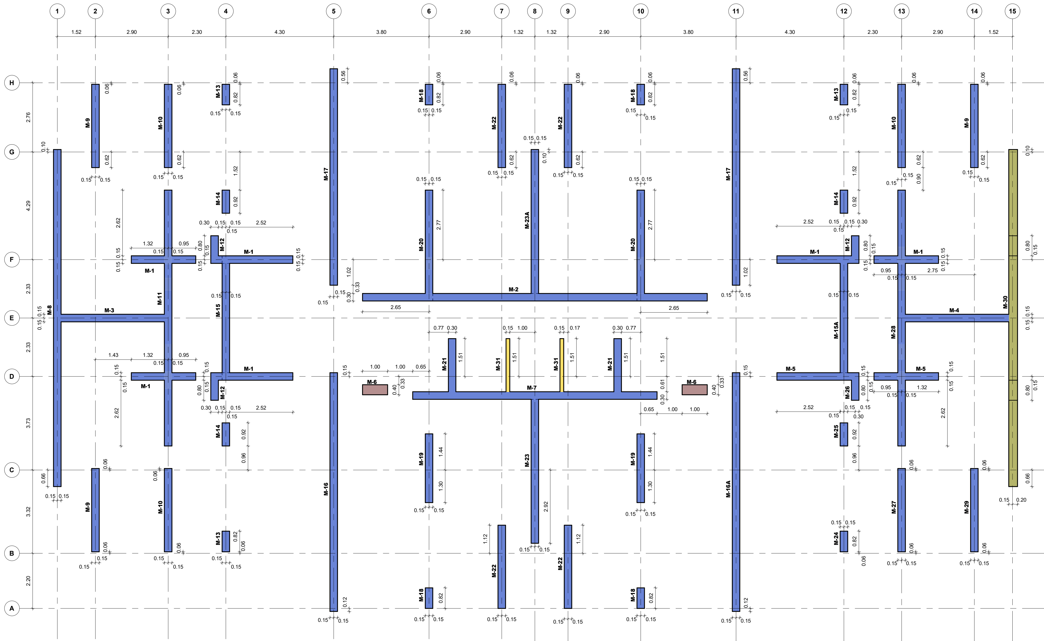
PLANTA LOCALIZACIÓN DE MUROS PISO TIPO 1 (PISO 3 A PISO 14) Escala 1 : 75
