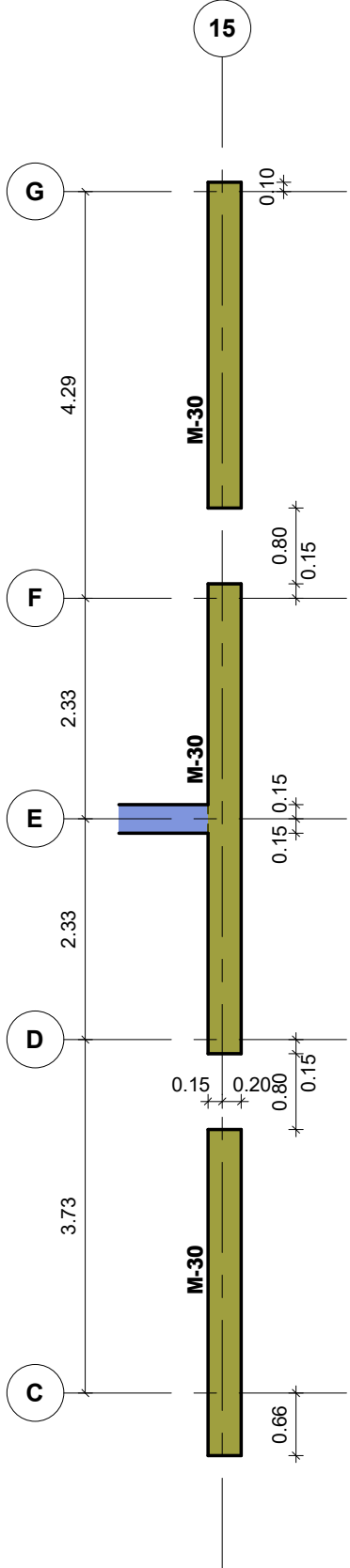
PLANTA LOCALIZACIÓN DE MURO M-30 PISO 7 A 14 Escala 1 : 75
